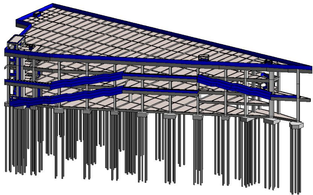
图 4 体育馆主体结构 (变更前) 模型示意图
