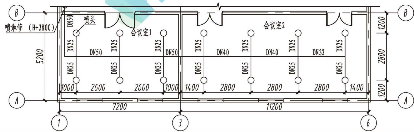
喷淋系统平面图 1:100
