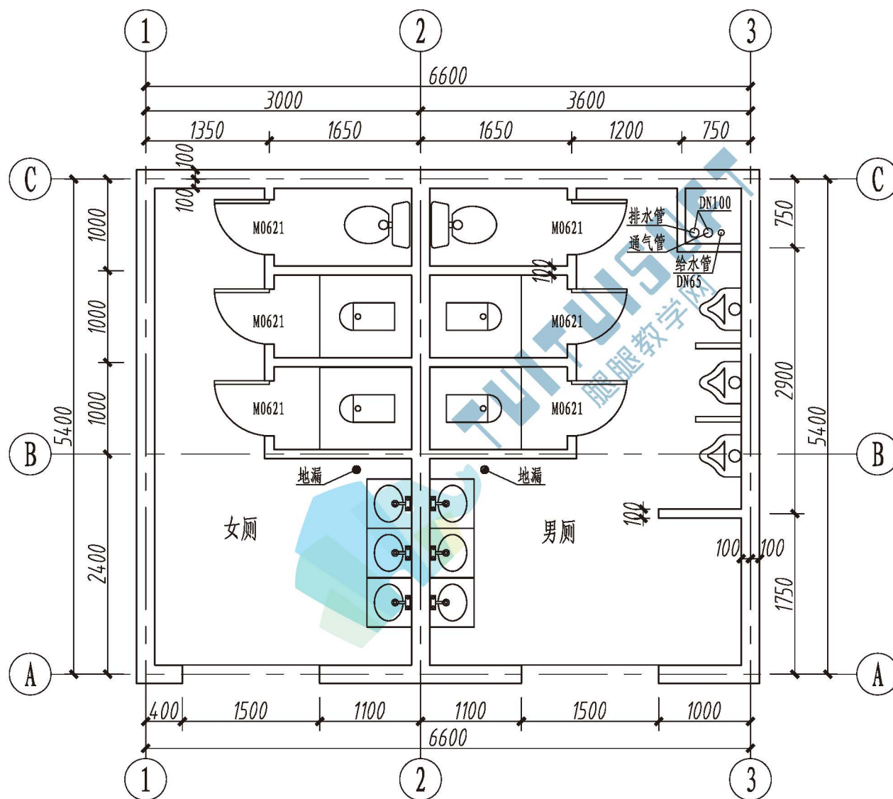
平面图 1:50
